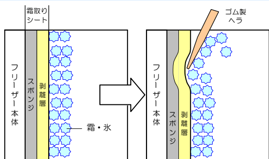
フリーザー内部取付例
