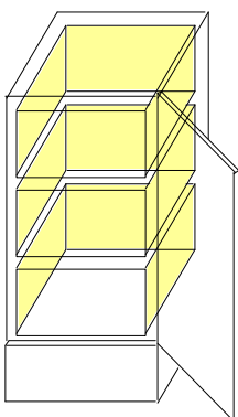
フリーザー内部取付例
